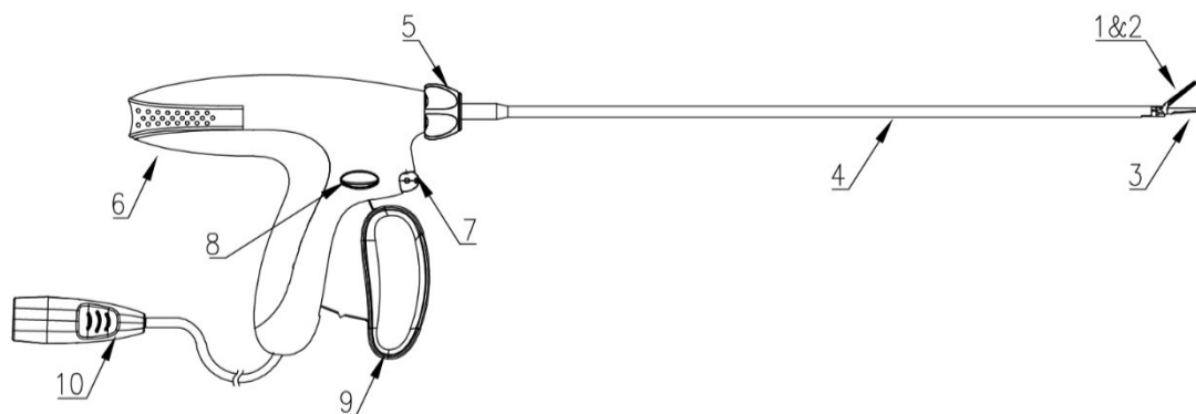
图 1.11 一次性使用超声软组织刀头 SASD23L/SASD36L/SASD45L
