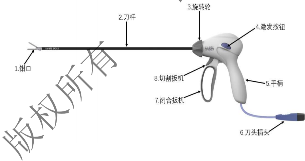
图 1.13 一次性使用高频切割闭合器械
