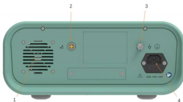
图 1.3 发生器后面板
