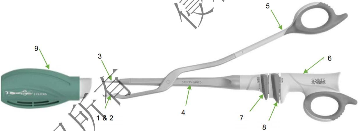
一次性使用超声软组织手术刀头 SASG17F
