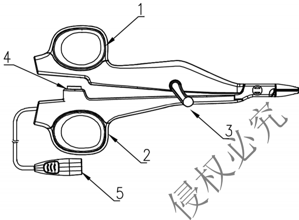
图1.17 一次性使用超声高频切割闭合器械SPSE12/SPSE12T/SPSE19/SPSE19T
